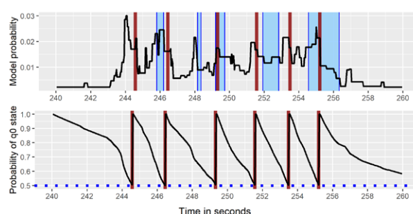
Figure 2 : Le modèle calcule la probabilité de feedback (représentée par la courbe noire dans le panneau supérieur) et prédit un feedback lorsque cette probabilité dépasse un seuil spécifique (indiqué par la ligne rouge verticale). Le feedback prédit est comparé au feedback observé (représenté par les zones bleues) pour évaluer la performance du modèle.
