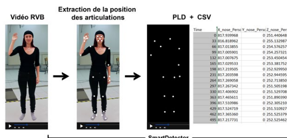
Figure 1 : Méthode proposée pour la génération de PLD avec SmartDetector
